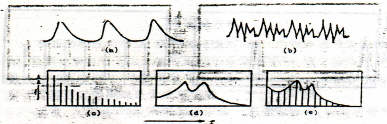
图 3.8 语音的声腔调节示意图: (a) 声带脉冲, (b) 幅射波, (c) 声带谱, (d) 声腔共振包络, (e) 语音频谱
