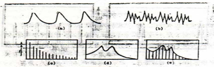
图 3.8 语音的声腔调节示意图: (a) 声带脉冲, (b) 辐射波, (c) 声带谱, (d) 声腔共振包络, (e) 语音频谱
